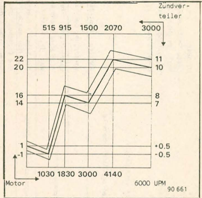
FLIEHKRAFT-VORZÜNDKURVE
